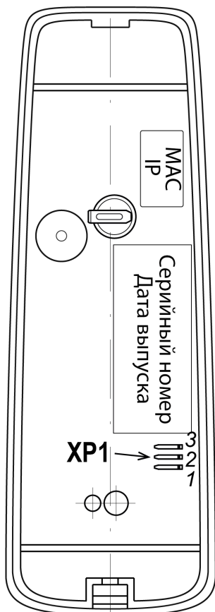
Рисунок 1. Внешний вид тыльной стороны контроллера
